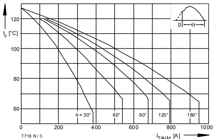
Bild / Fig. 3 Höchstzulässige Gehäusetemperatur / Max. allowable case temperature t_A = f(I_{TAVM}) Beidseitige Kühlung / Two-sided cooling Parameter: Stromflußwinkel / Current conduction angle \theta
